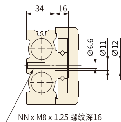
截面AA
